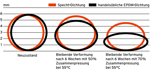
Vergleich der dauerhaften Verformung von Dichtprofilen (6 mm)
